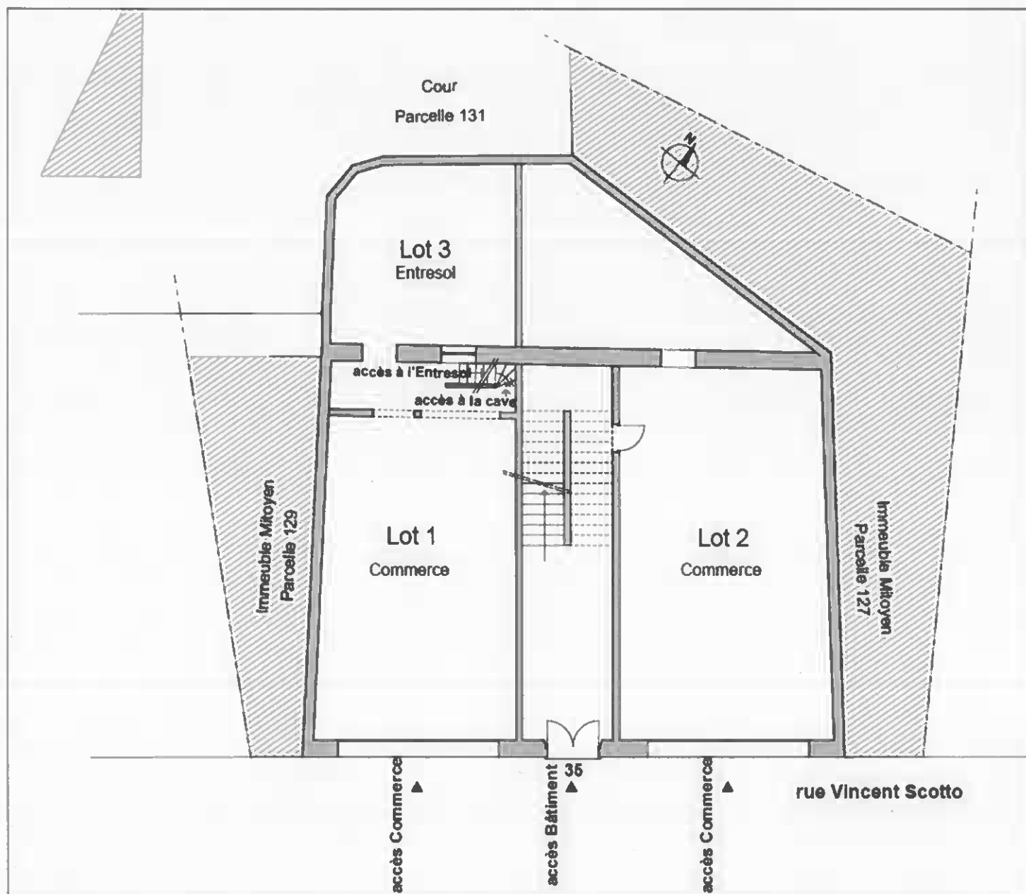
Plan RdC
